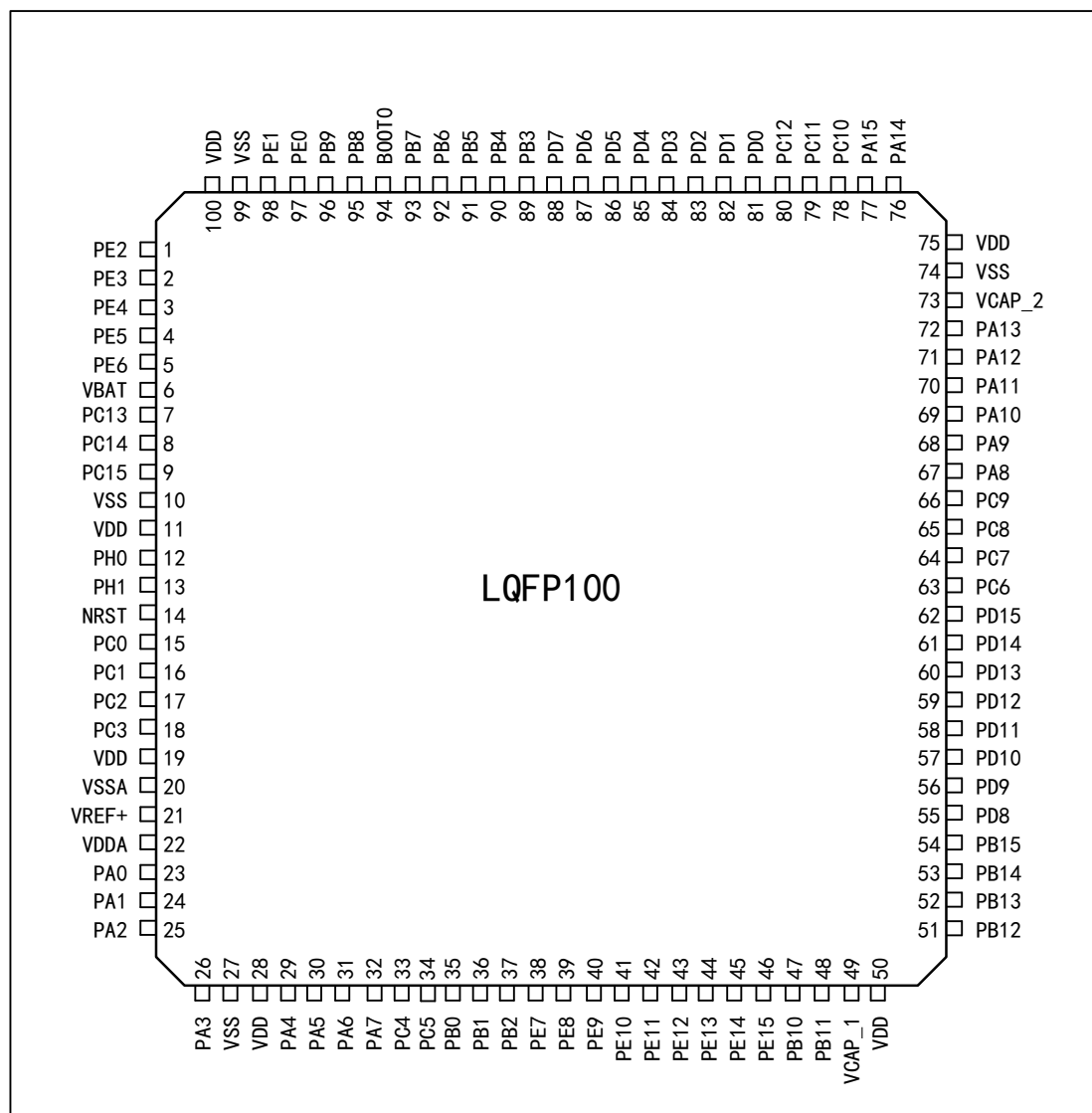
图 3 APM32F415xG 417xExG 系列 LQFP100 引脚分布图
