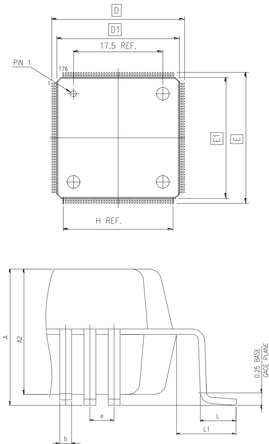
图 16 LQFP176 封装图
